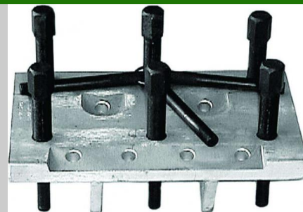
213 700 Estrattore 213 701 Bullone
