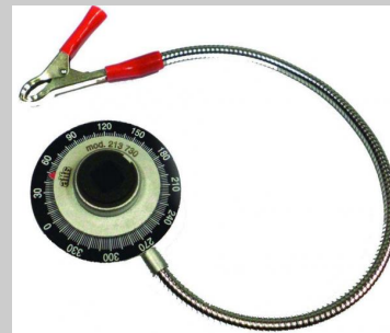
213 730 Att.1/2' - 2° 213 731 Att.3/4' - 2°
