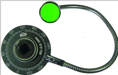
213 726 Att.1/2' - 2° 213 728 Att.3/4' - 2°
